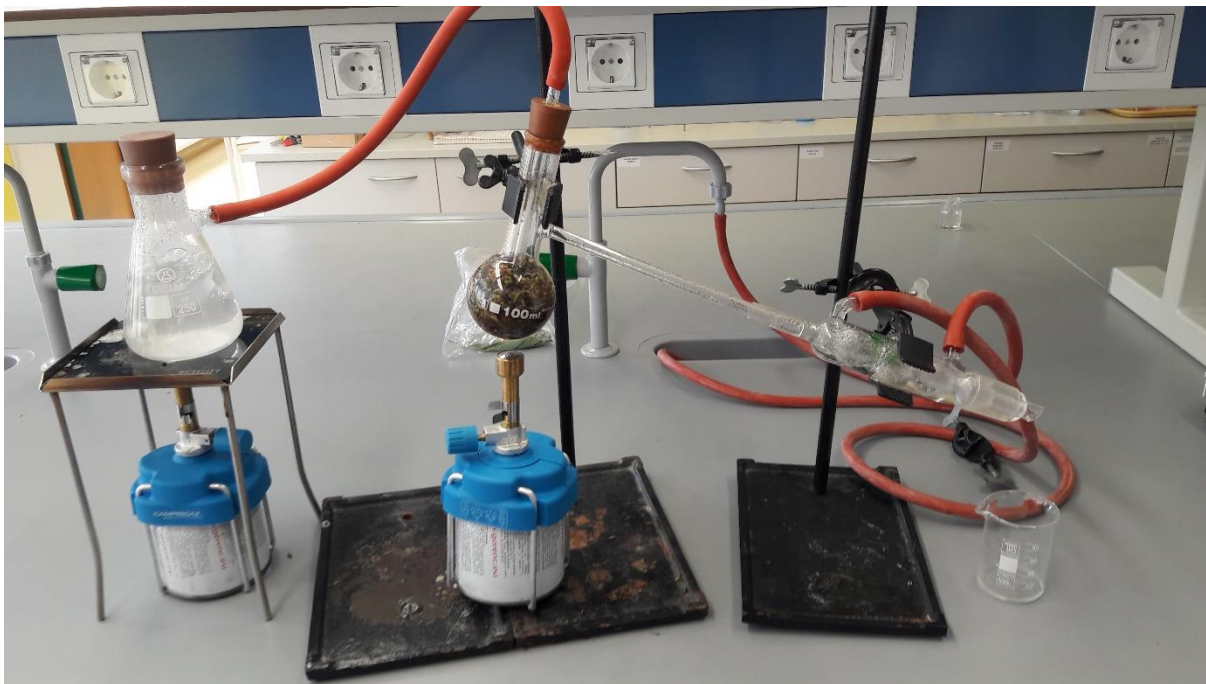
Destilacija eteričnega olja
